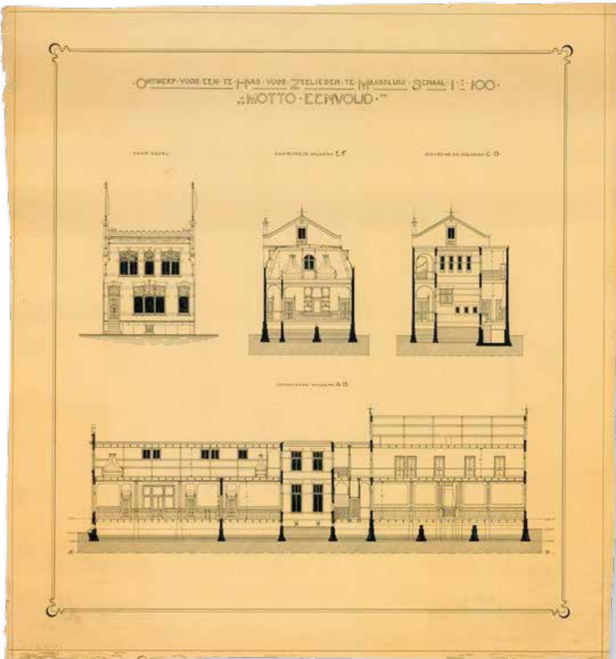
Een van de ingezonden bouwtekeningen voor een mogelijk Tehuis voor Zeelieden te Maassluis. Ingediend door architect Pieter Nicolaas Leguit (1874-1941).
