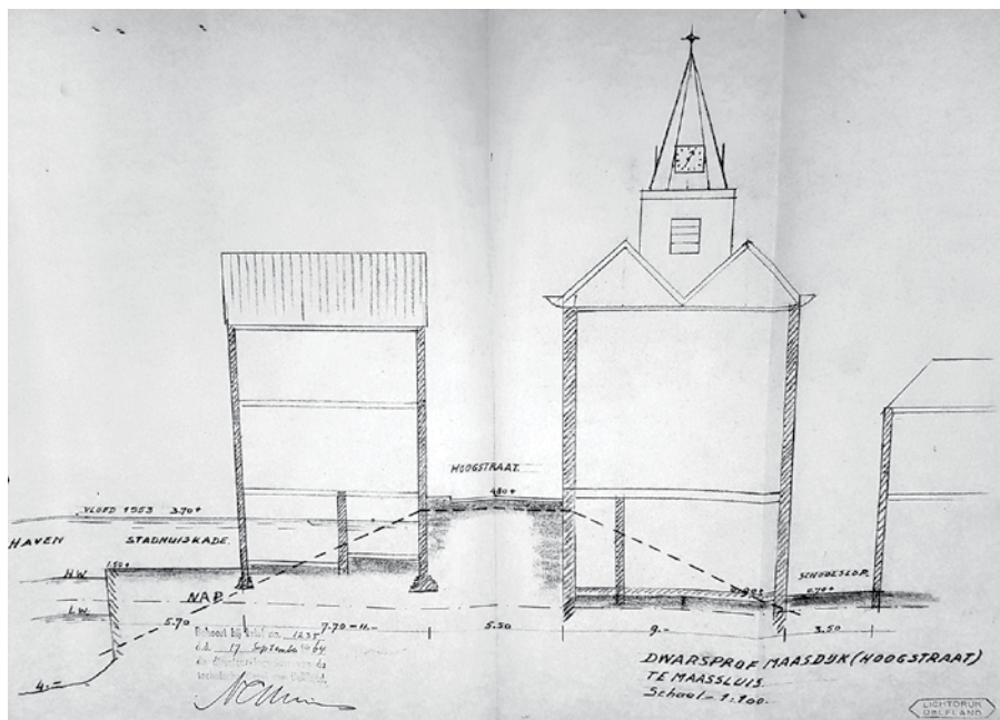
Dwarsdoorsnede van de Kleine Kerk. In de ruimte onder de kerkvloer was plaats voor twee verdiepingen.
